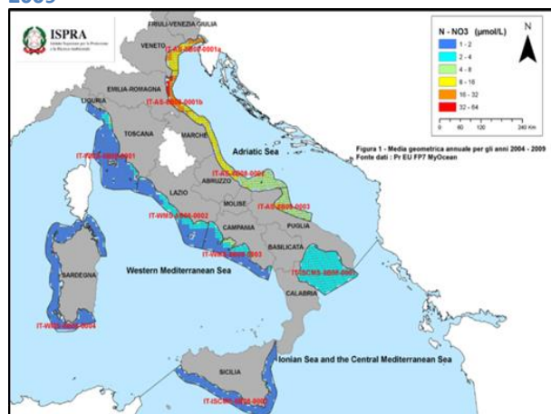
Figura 96 Andamento spaziale della concentrazione di Nitrati Media geometrica annuale nel periodo 2004-2009
