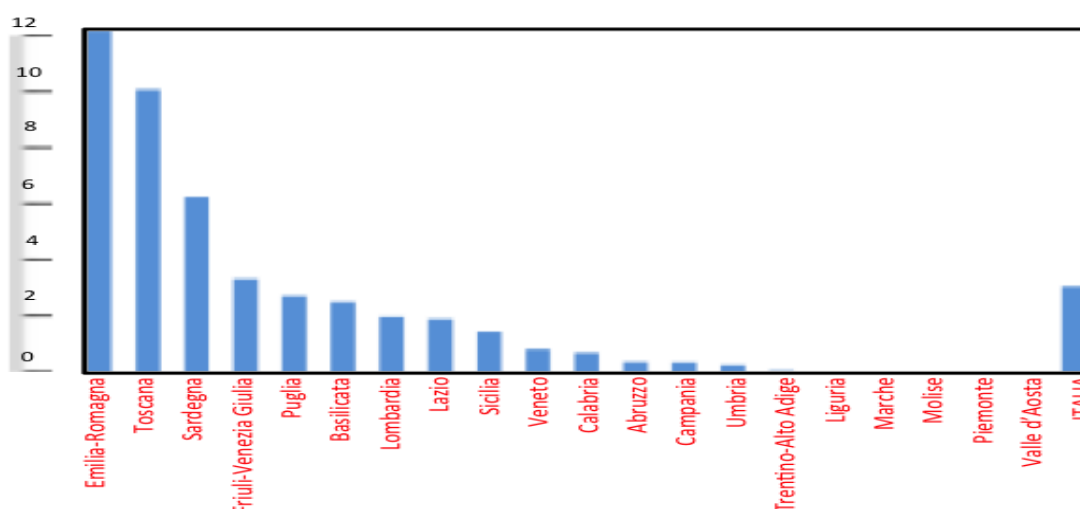
Figura 42 Zone umide di importanza internazionale: millesimi di superficie regionale occupata da aree Ramsar
