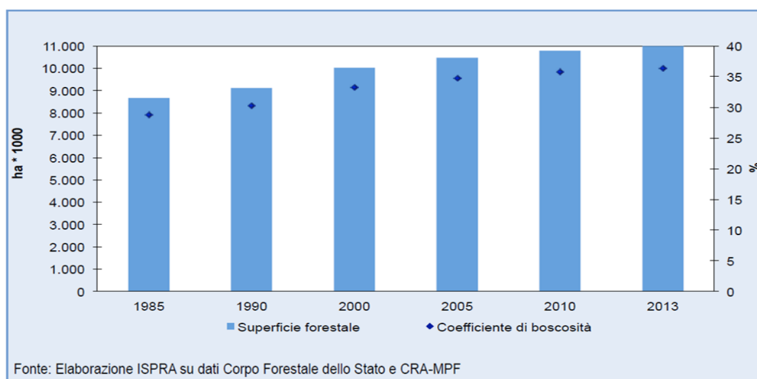
Figura 105 Andamenti di superficie forestale coefficiente di boscosità in Italia.
