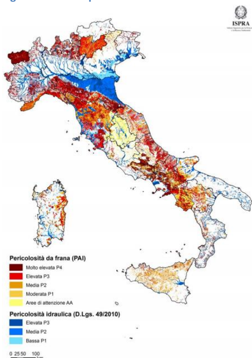
Figura 90: Aree a pericolosità da frana e idraulica
